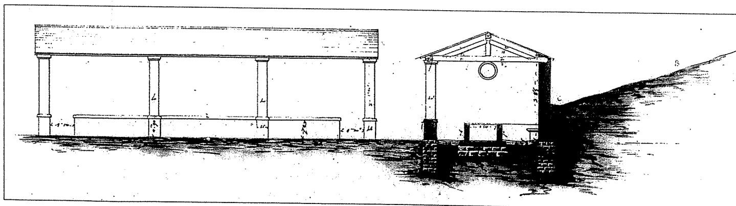
Plan, vue frontale et coupe du nouveau lavoir à construire.
